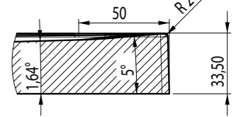
DETAIL B MAßSTAB 1:2
