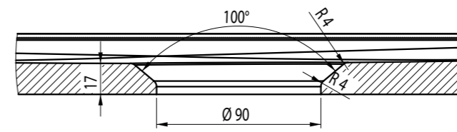
DETAIL D MAßSTAB 1:2
